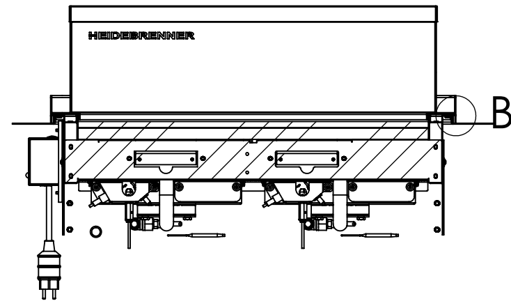
SCHNITT A-A
