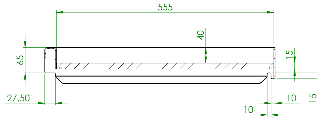
SCHNITT A-A
